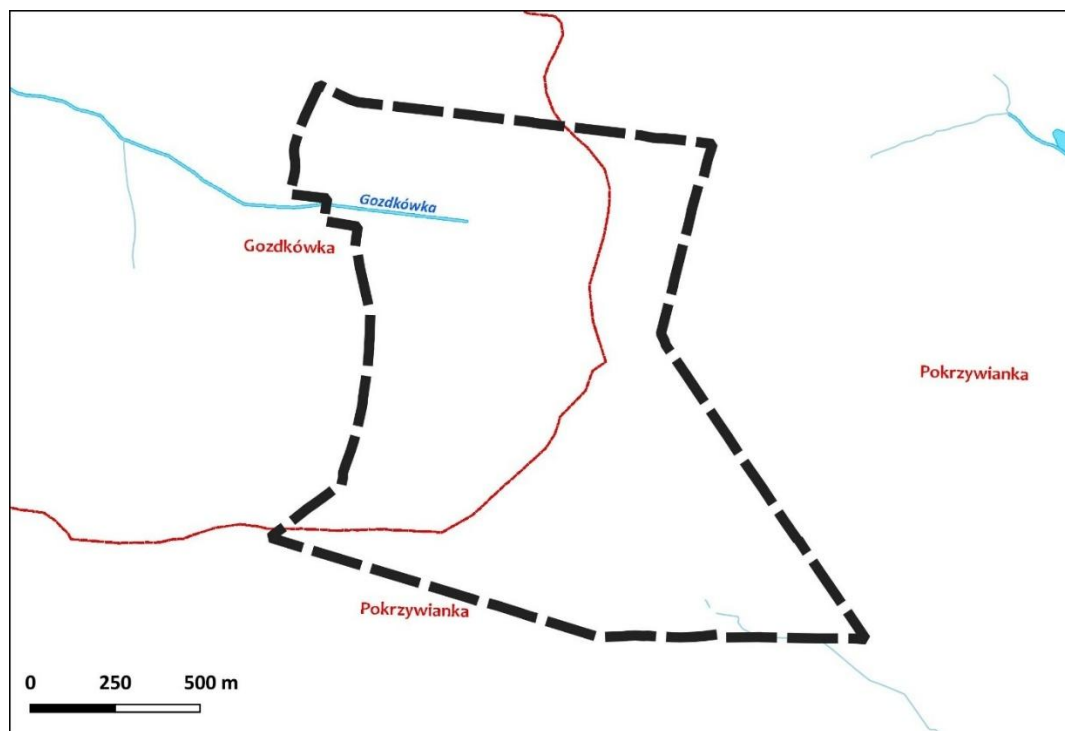
Rysunek 6. Zlewnie poziomu 6 na terenie opracowania
